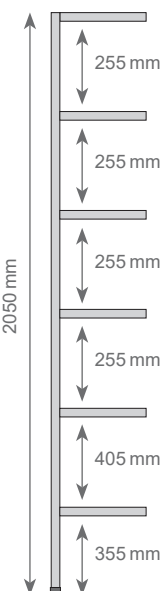
Altura 2050 mm / 6 niveles Height 2050 mm / 6 levels Hauteur 2050 mm / 6 niveaux Höhe 2050 mm / 6 Ebenen
